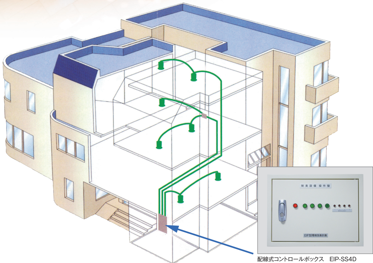
配線式コントロールボックス EIP-SS4D
