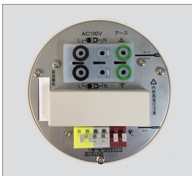
天板（電気接続部）
